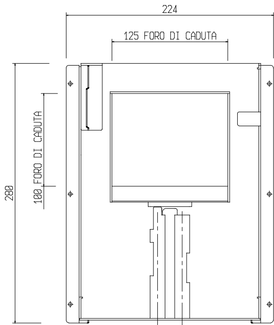
PIASTRA GUIDA SACCO
